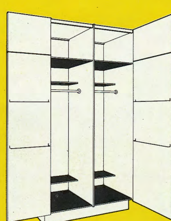
VAATEKOMERO 4218 K 4219 K lev. 98 cm 118 cm
